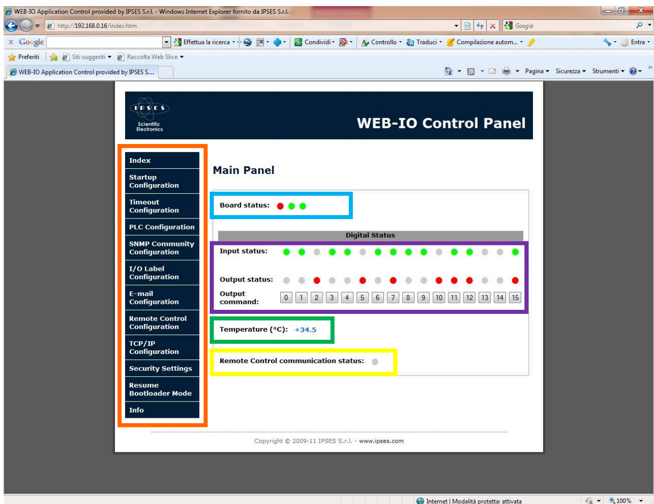
Figura 7: Pagina principale server http .
