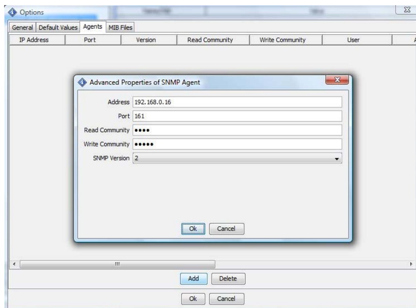
Figura 21: MIB browser e configurazione dell'Agent SNMP.
