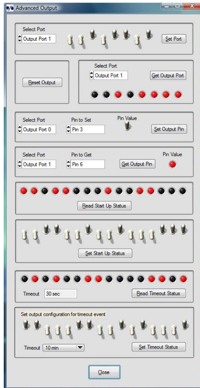
Figura 25: finestra avanzata di opzioni uscita.
