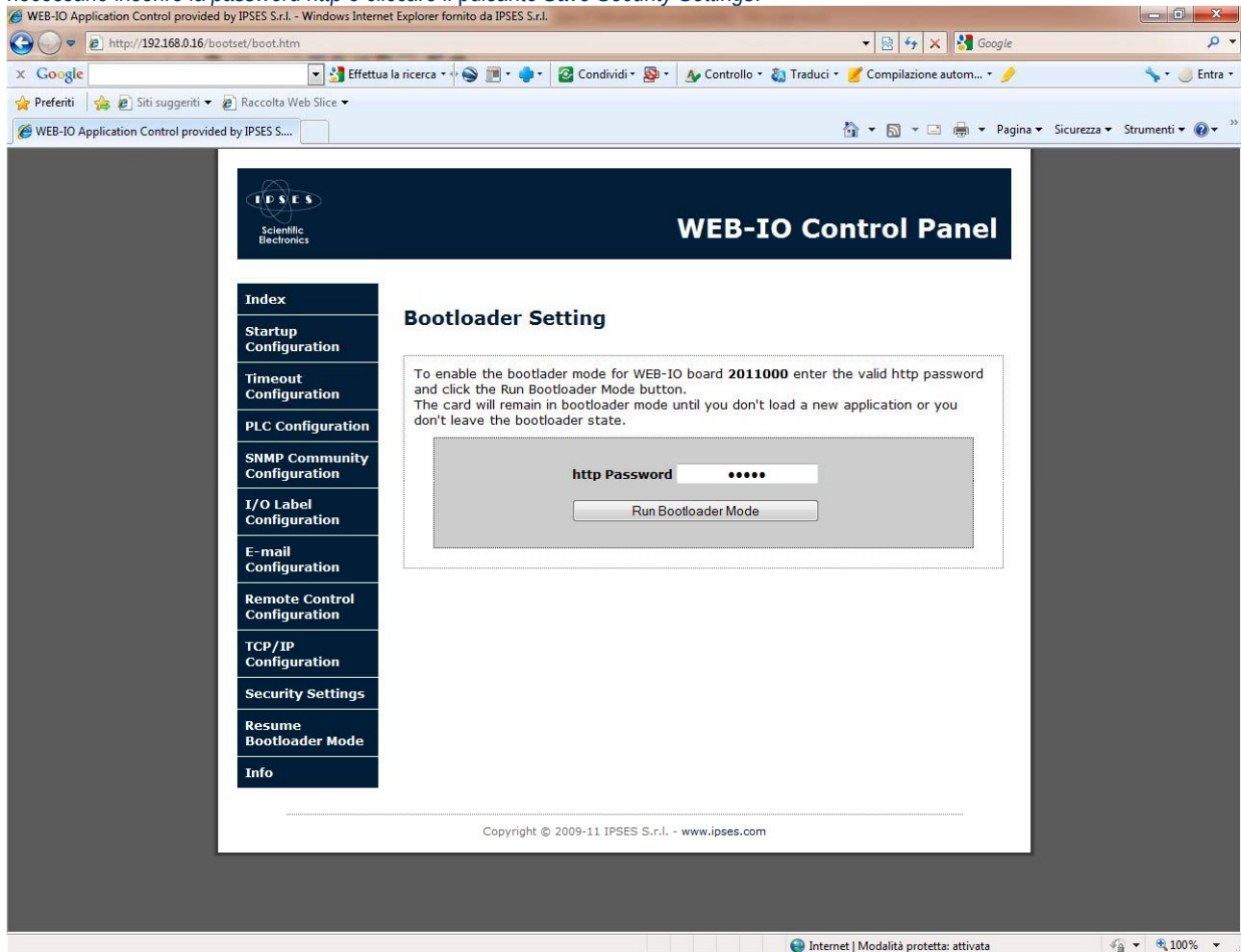
Figura 17: Pagina di accesso alla modalità Bootloader.
