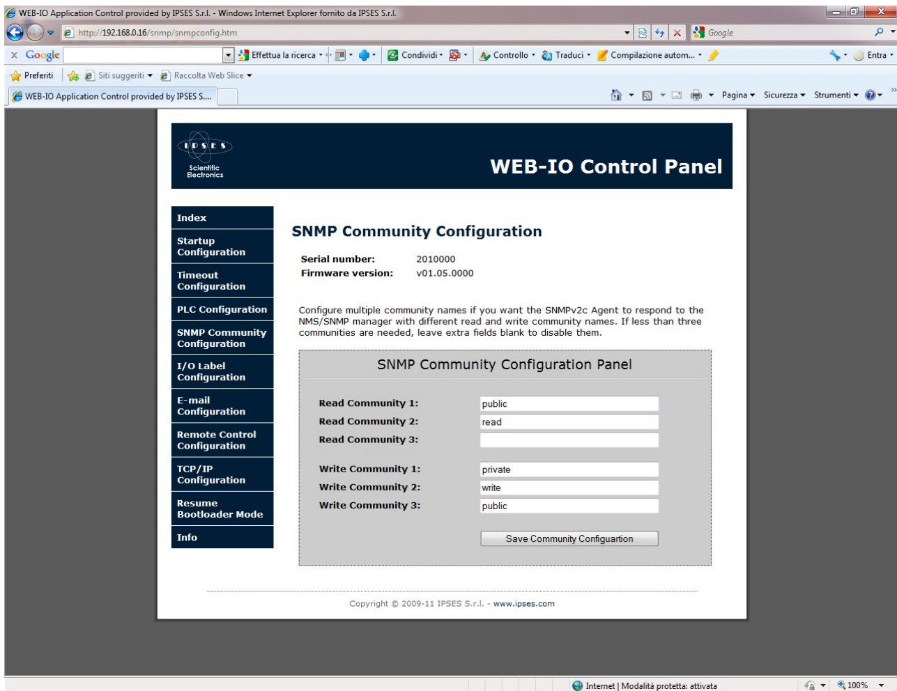
Figura 11: Pagina di configurazione delle Community SNMP.
