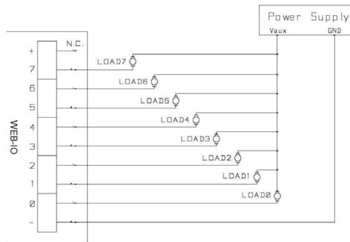
Figura 4a: schema elettrico di connessione delle uscite.
