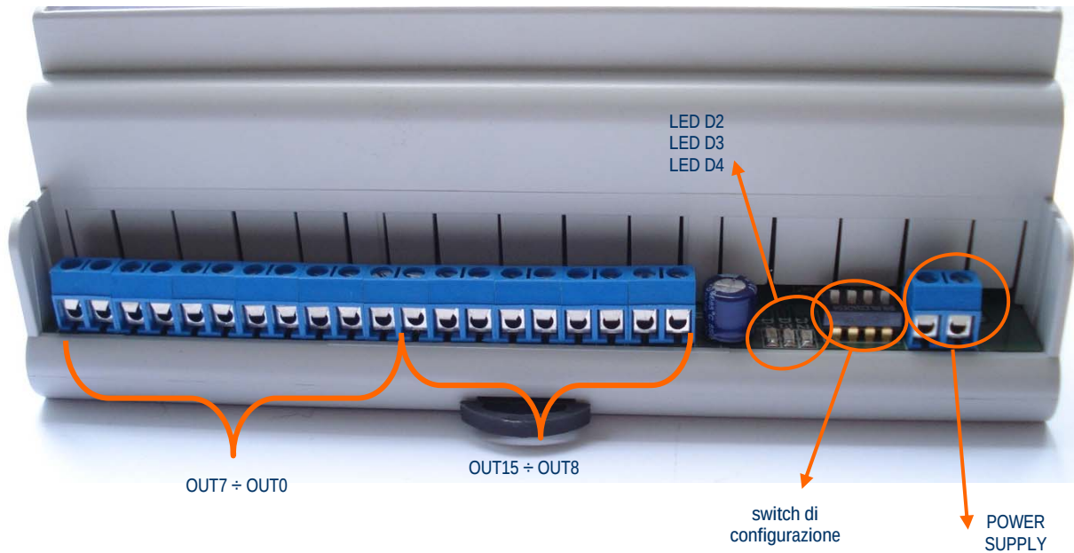
Figura 3: WEB-IO BOX lato con gli output e gli switch di configurazione
