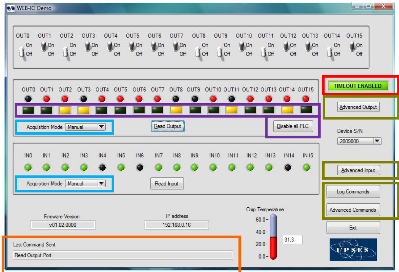
Figura 23a: finestra principale del software demo.
