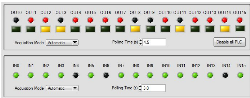
Figura 23b: acquisizione automatica degli ingressi e delle uscite.
