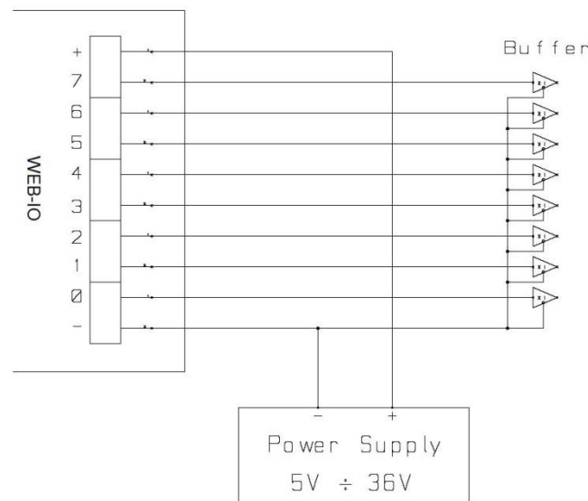
Figura 4b: schema elettrico di connessione delle uscite.
