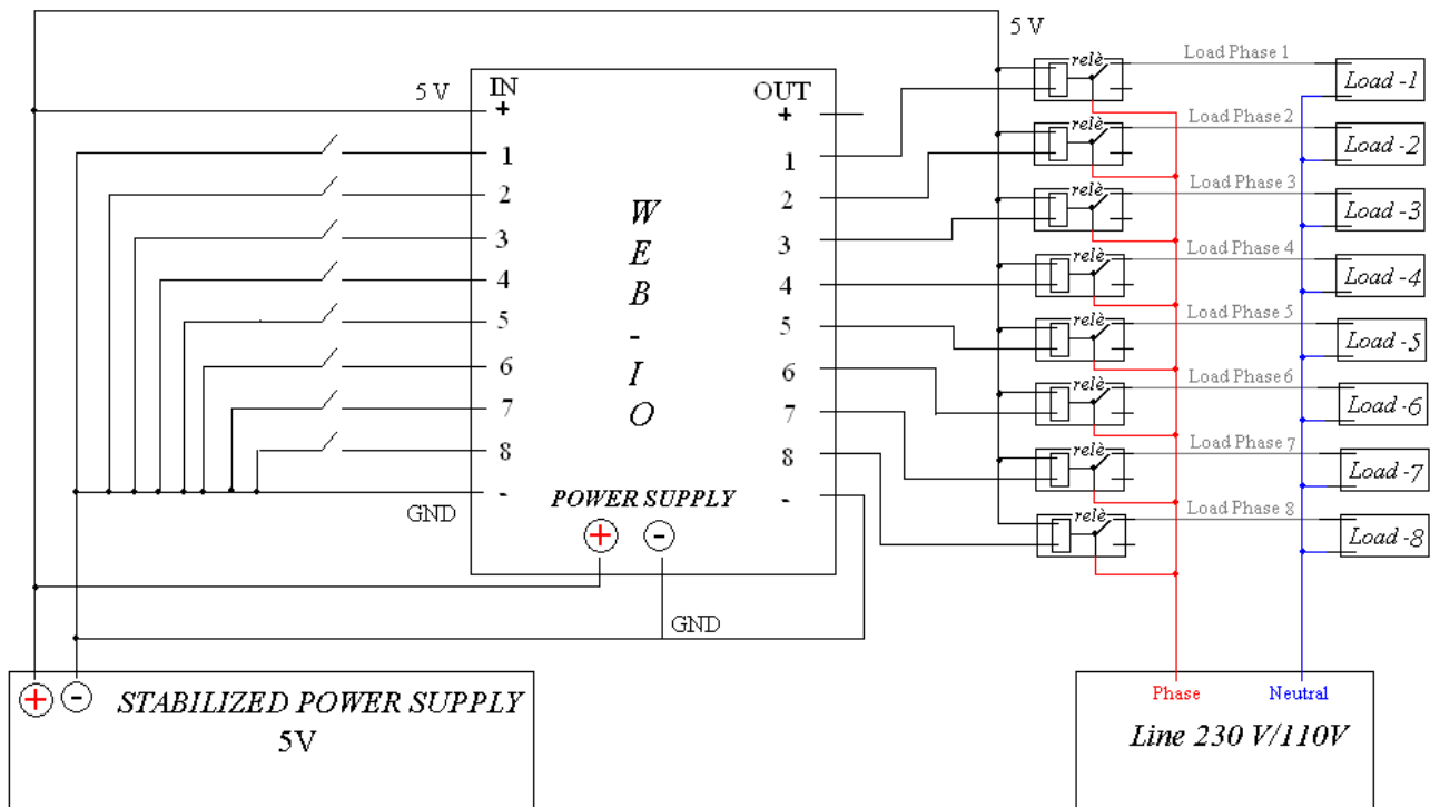
Figura 6: controllo del carico esterno con alimentazione da rete
