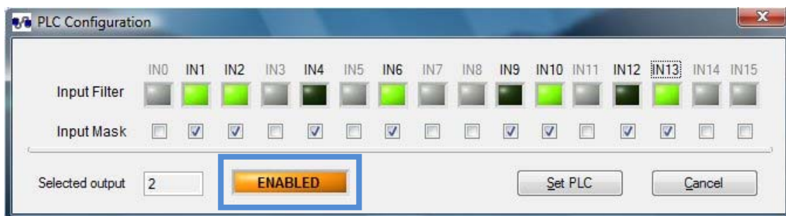
Figura 24: finestra di pop-up per la configurazione dei parametri di maschera e filtro PLC.
