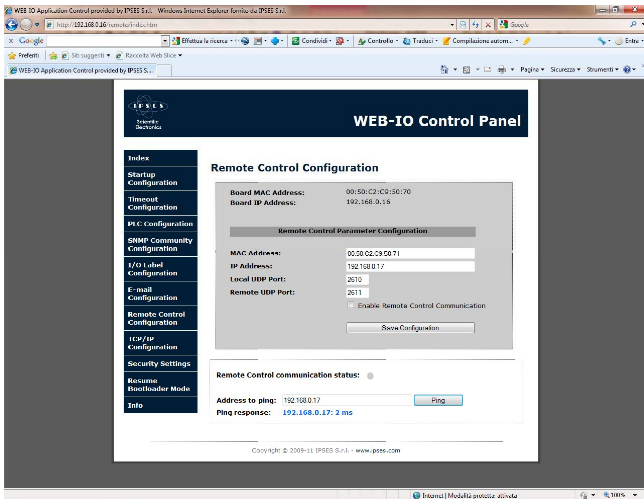
Figura 14: Pagina di configurazione dei parametri del servizio Remote Control .
