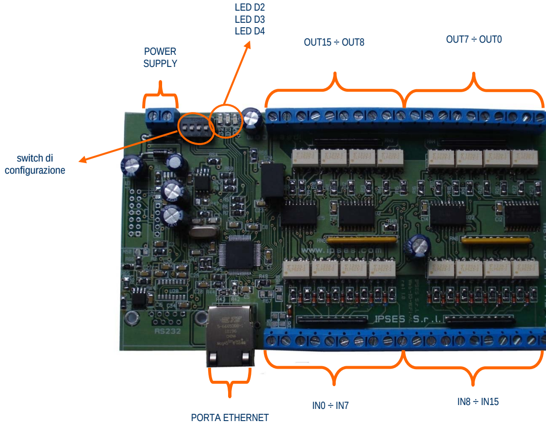
Figura 1: scheda WEB-IO BOX
