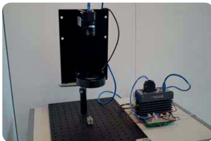
Figura 1: Architettura del sistema: Il sistema in laboratorio con la telecamera, il Compact Vision System, l'illuminatore configurato prima del montaggio
