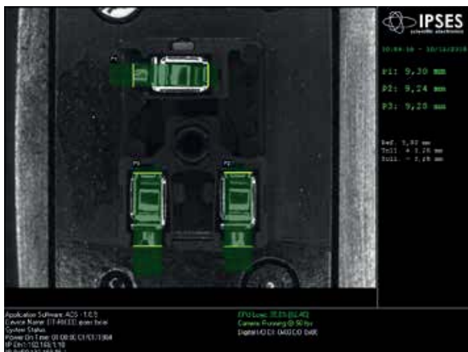
Figura 2: Interfaccia operatore: l'interfaccia operatore con l'esito delle misure e lo stato del sistema
